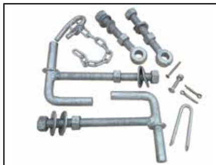
Vnr. 59031: Komplette beslagpakke til montering av lettvektsgrind på stolper.
